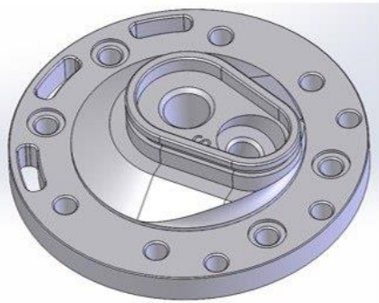
Твердотельная модель
