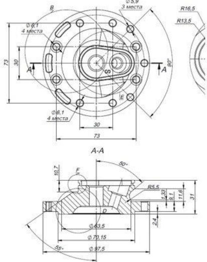
Чертеж
